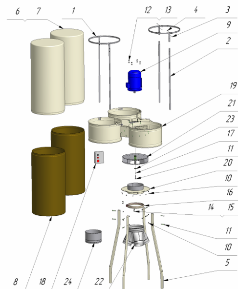
Комплектация УВП-М 5000К
