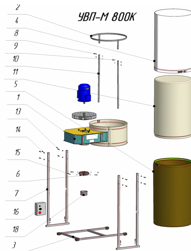
Комплектация УВП-М 800К
